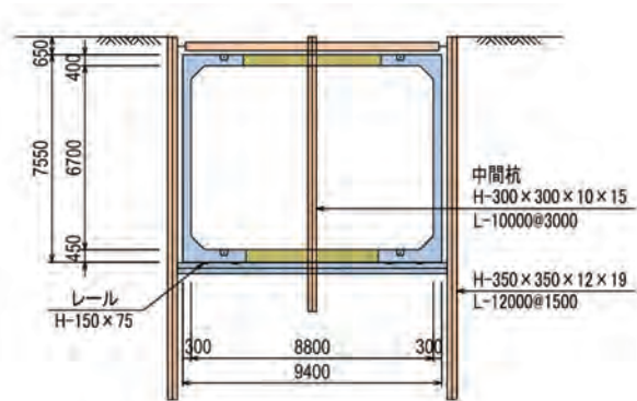
山留内施工断面図
