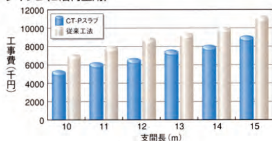
タイプB (B活荷重用)
