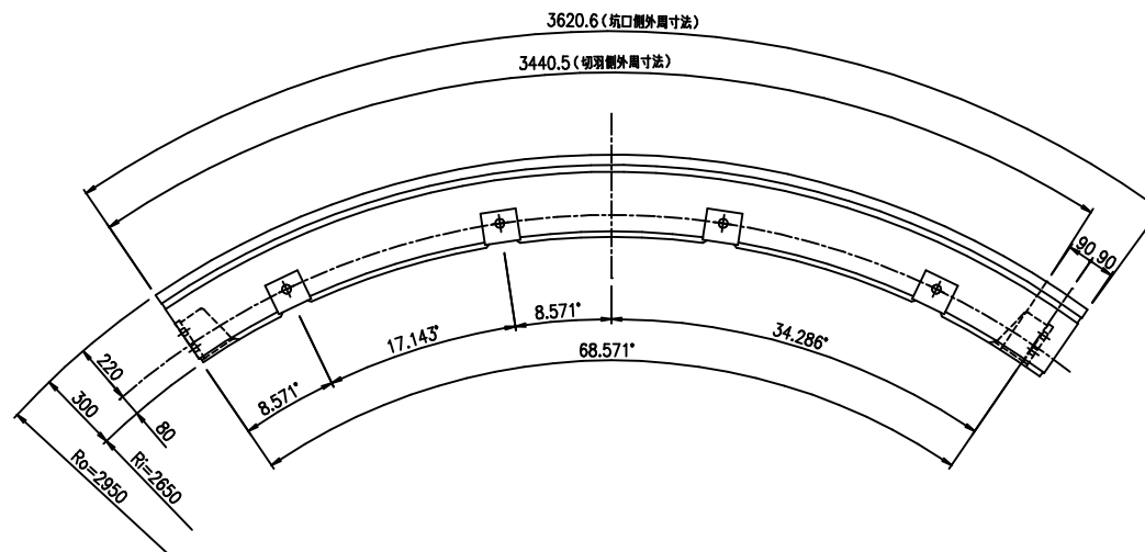
B1型セグメント S=1/15
