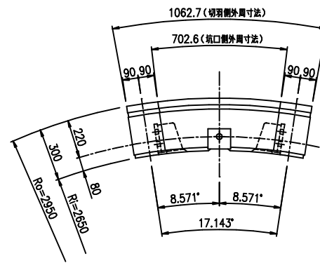
K型セグメント S=1/15
