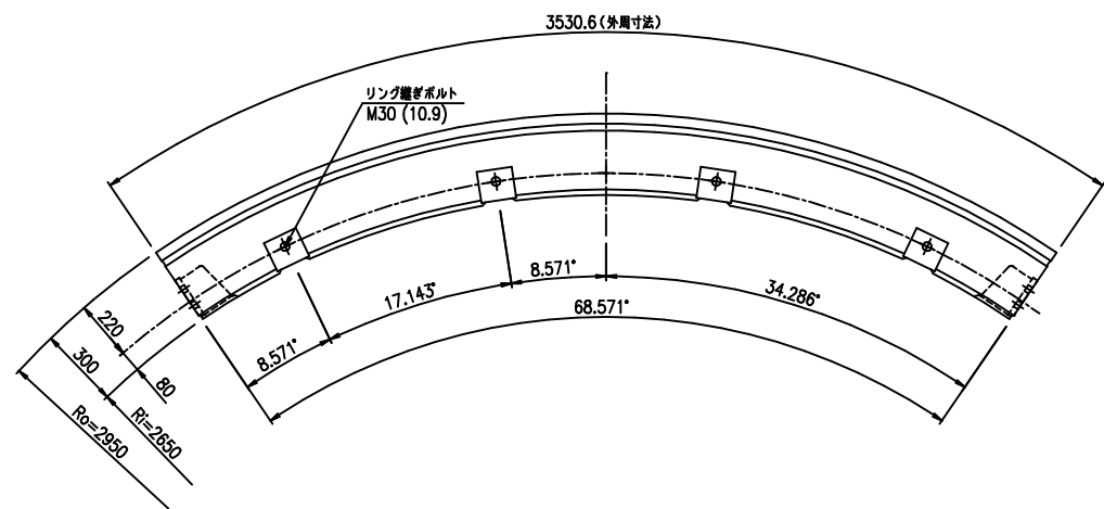
A型セグメント S=1/15
