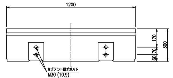
A-A S=1/10
