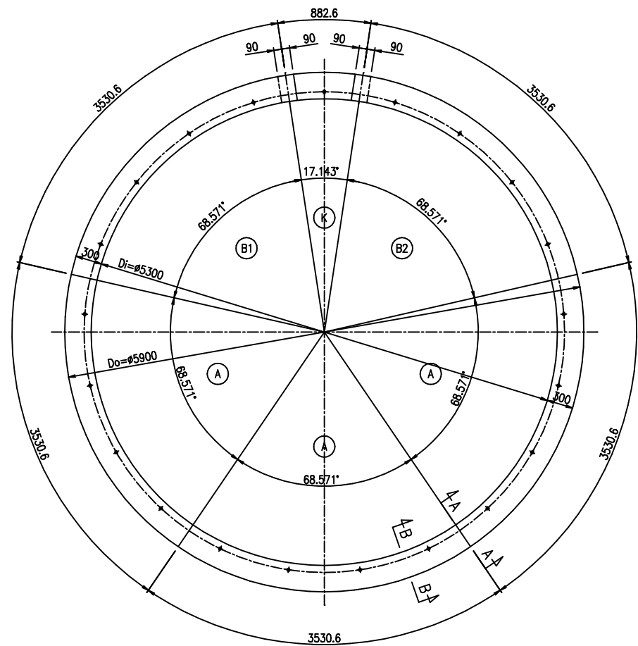
A型セグメント S=1/15
